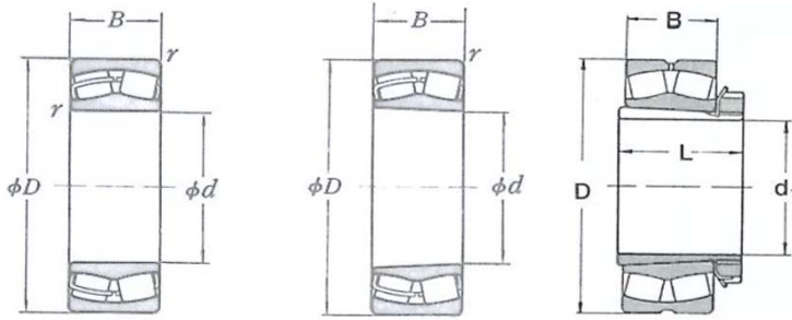
FURO CILÍNDRICO
